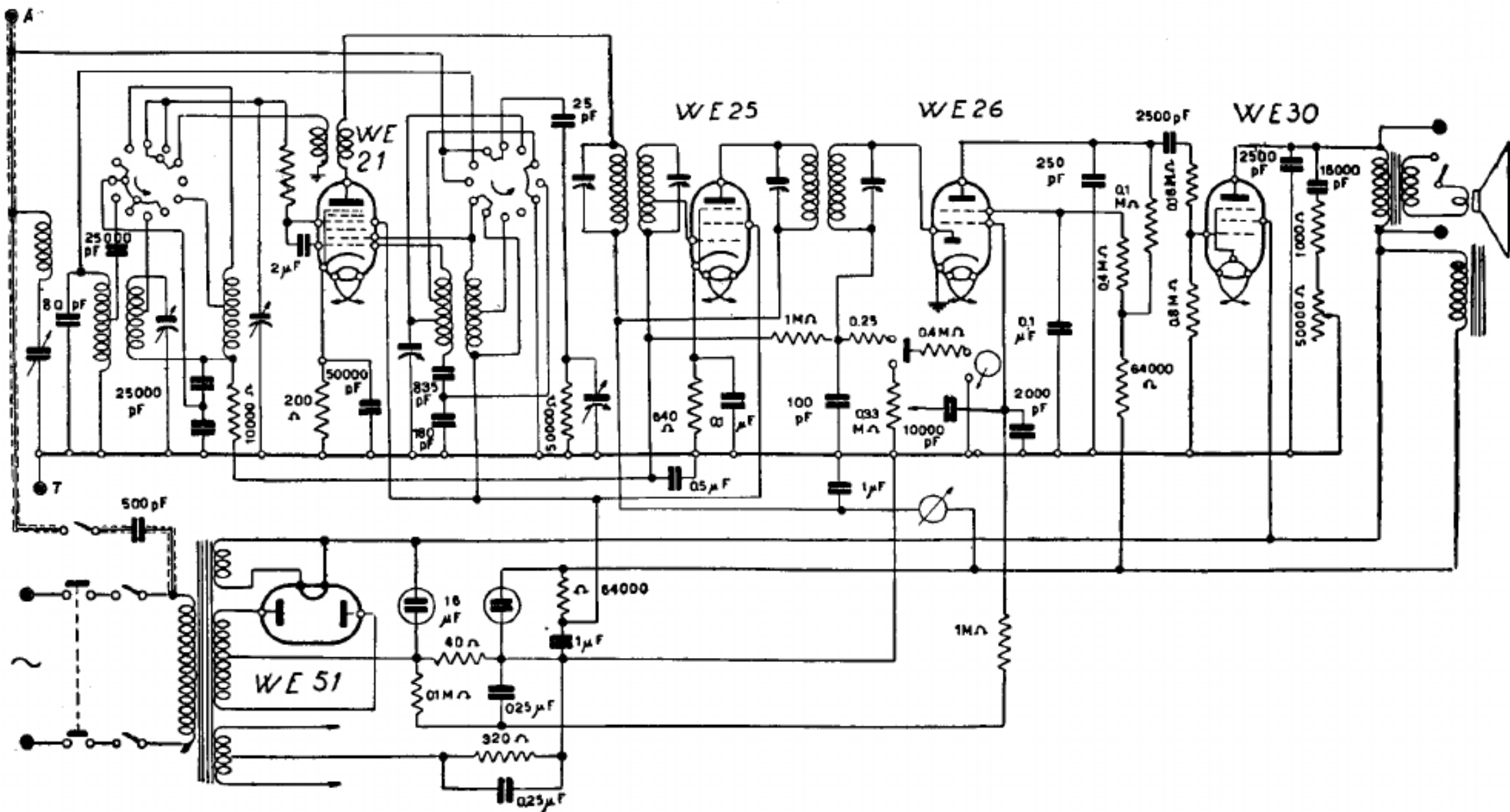
PHILIPS RADIO. — Mod. « 428 » e anche « 651 M, 653 M ». — (SUPER POPE P97A). — Media frequenza: 468 kHz. — Potenza: 3 W. — Produzione: 1935-1936.
